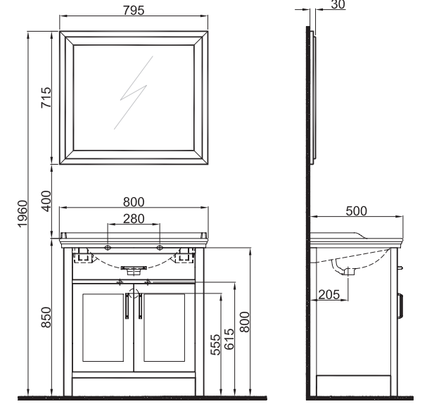
80 cm Setler Ön ve Yan Görünüş
