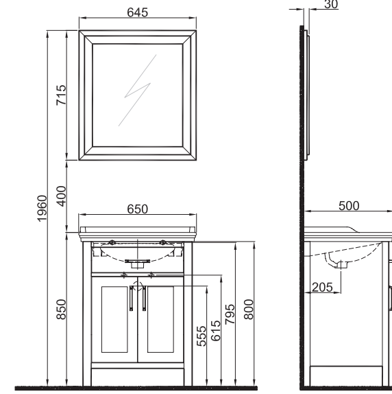
65 cm Setler Ön ve Yan Görünüş
