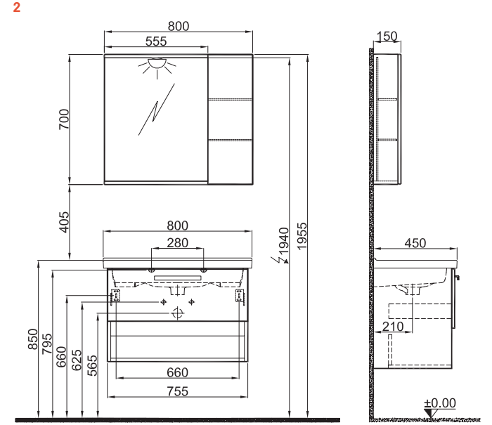
80 cm Set Ön ve Yan Görünüş
