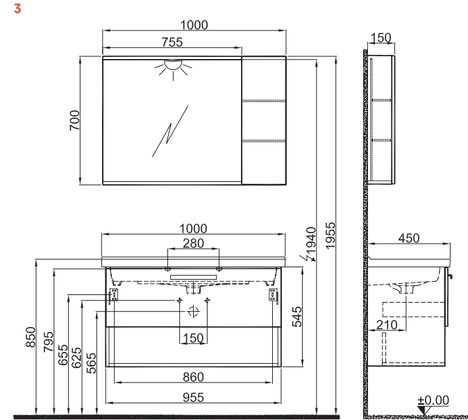
100 cm Set Ön ve Yan Görünüş
