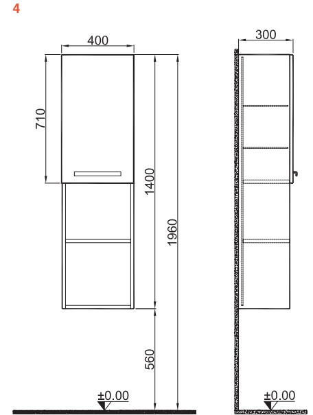
40 cm Boy Dolap Ön ve Yan Görünüş
