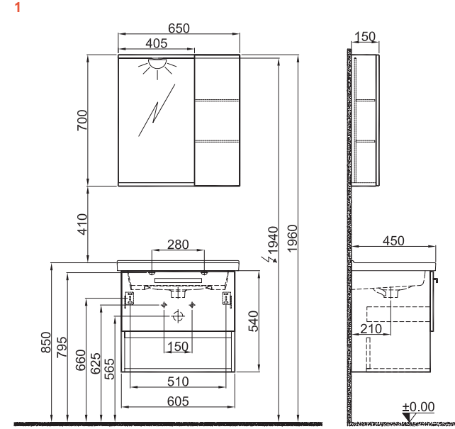
65 cm Set Ön ve Yan Görünüş
