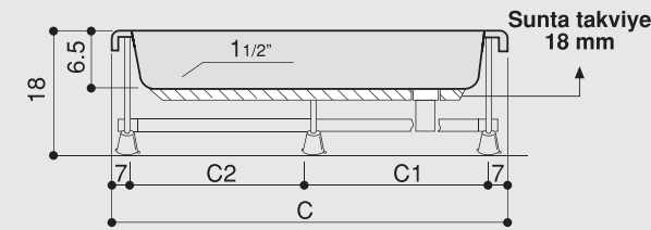
Kesit A-A
