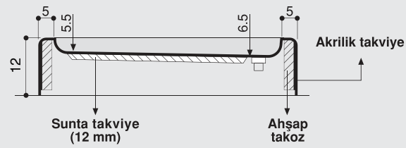
Kesit A-A
